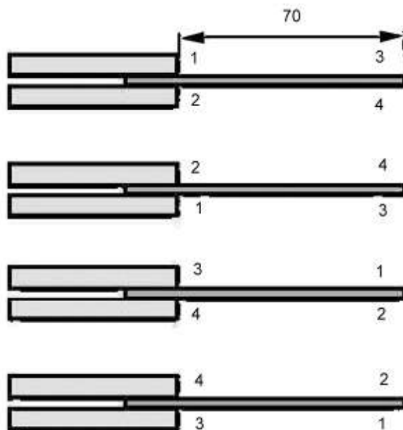
Рисунок 2 – Положения зажима образца ленты
