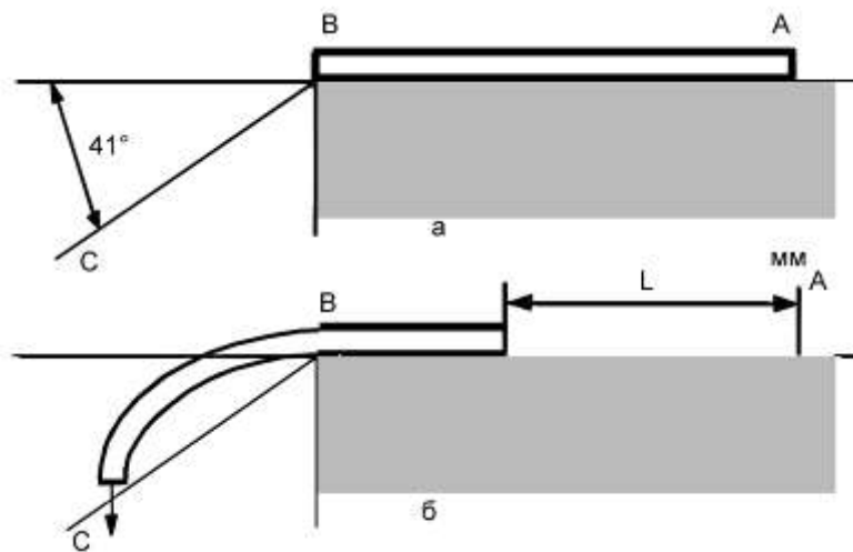
Рисунок 5 – Схема определения жесткости фала
