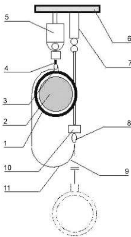
Рисунок 7 – Схема установки для испытания пояса при воздействии динамической нагрузки
