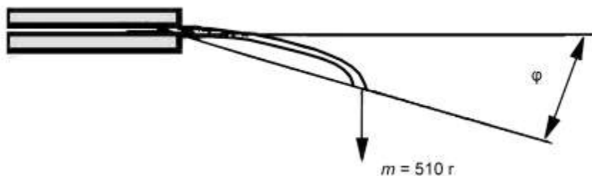
Рисунок 3 – Схема измерения угла сгиба
