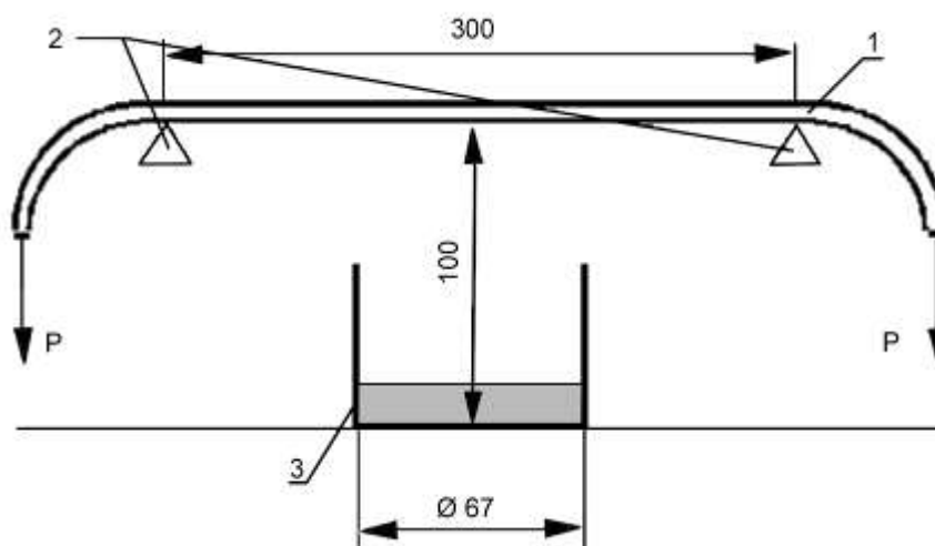
1 – образец фала; 2 – опоры; 3 – емкость для спирта
